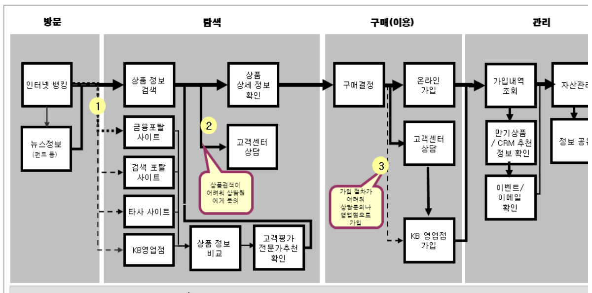
[그림 1-11] 다이어그램 버전의 시나리오 작성 예시 3: 각 단계별로 어떤 구체적인 흐름으로 전개되는지 확인할 수 있는 도식
